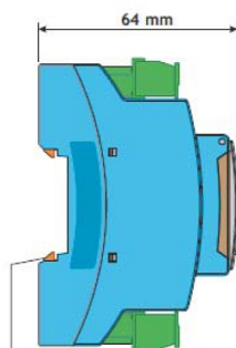
Montage auf Hut-Schiene gem. DIN EN50022
