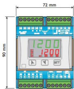
Abnehmbare Klemmenanschlüsse
